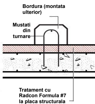
DETALIU RM1 Bordura
