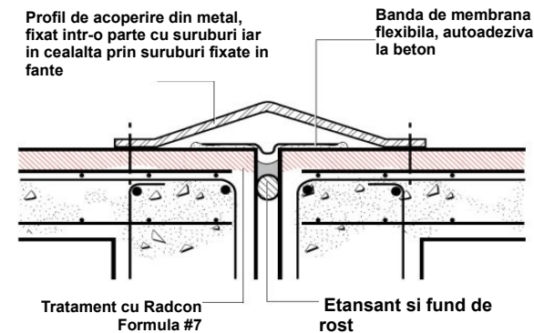
DETALIU REJ3 Rost de dilatare
