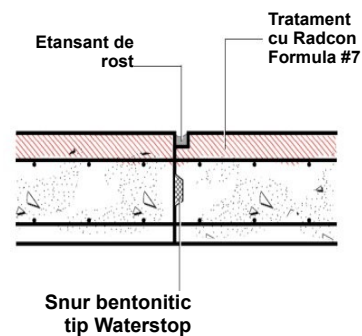
DETALIU RPJ2 Rost de constructie
