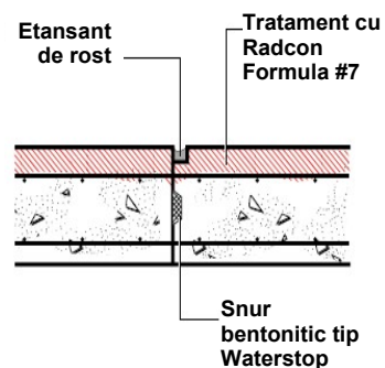
DETALIU RPJ2 Rost de constructie
