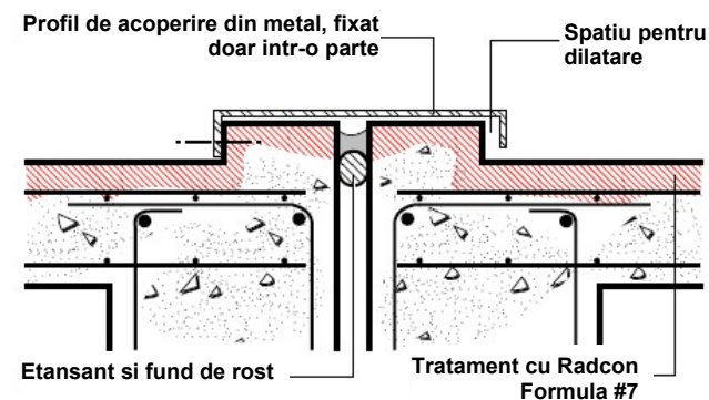
DETALIU REJ2 Rost de dilatare
