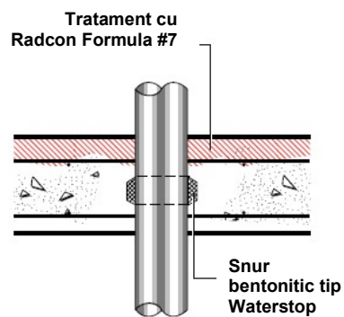
DETALIU RP1 Strapungere
