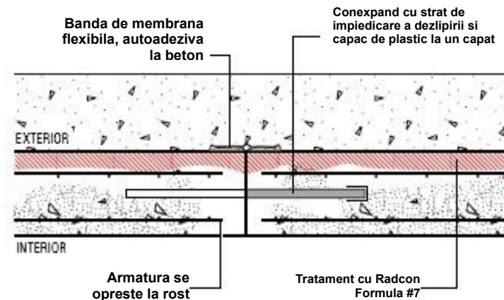
DETALIU TCJ1 Rost de contractie
