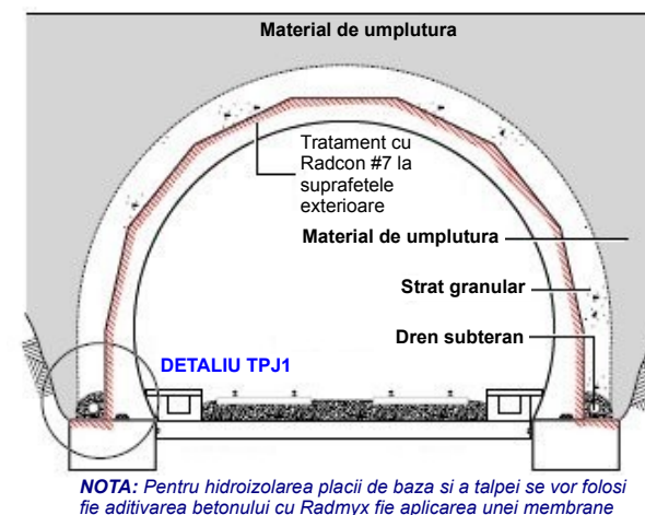
SECTIUNE TIPICA PRINTR-UN TUNEL FERROVIAR
