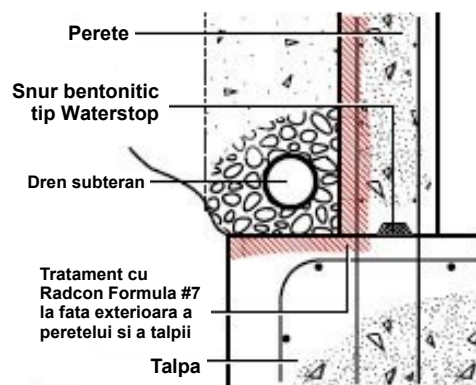
DETALIU TPJ1 Rost de constructie
