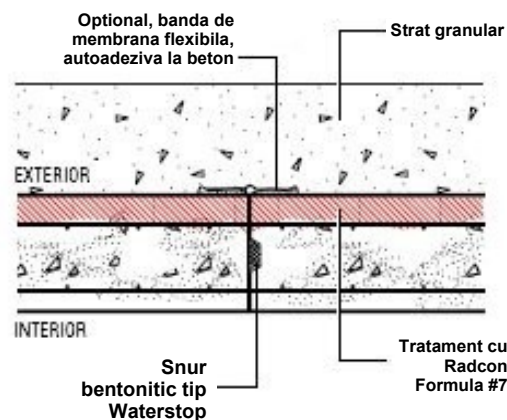
DETALIU TPJ2 Rost de constructie
