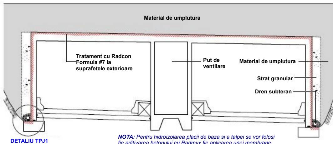
SECTIUNE TIPICA PRINTR-UN TUNEL RUTIER
