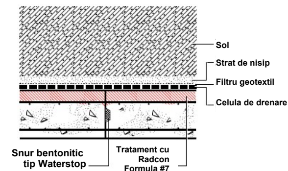
DETALIU RPJ1 Rost de constructie
