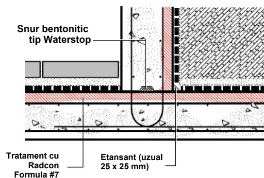
DETALIU RPJ5 Rost de constructie
