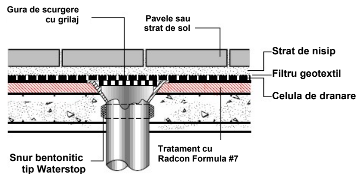
DETALIU RP3 Strapungere
