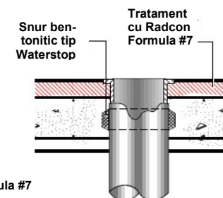
DETALIU WP1 Strapungere
