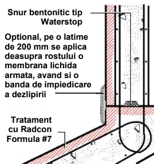
DETALIU WPJ4 Rost de construcție
