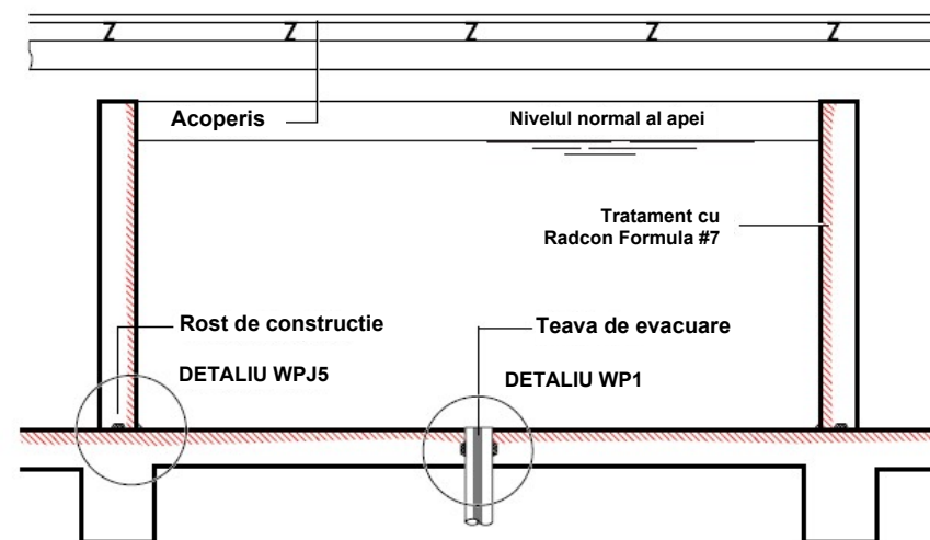
SECȚIUNE TIPICĂ PRINTR-UN TURN DE APA, tip SPRINKLER
