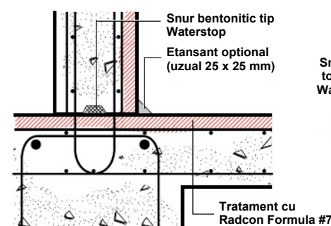
DETALIU WPJ6 Rost de construcție
