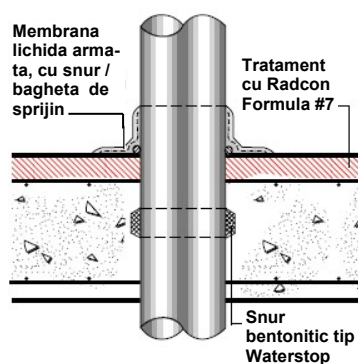
DETALIU WP4 Strapungere
