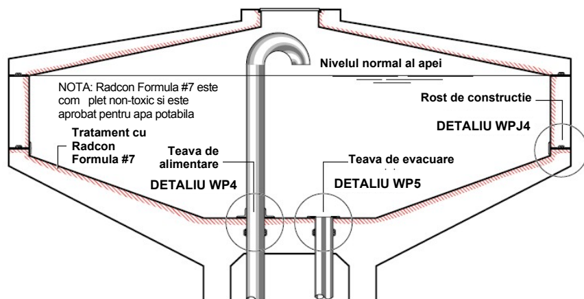
SECȚIUNE TIPICĂ PRINTR-UN TURN DE APA SUSPENDAT
