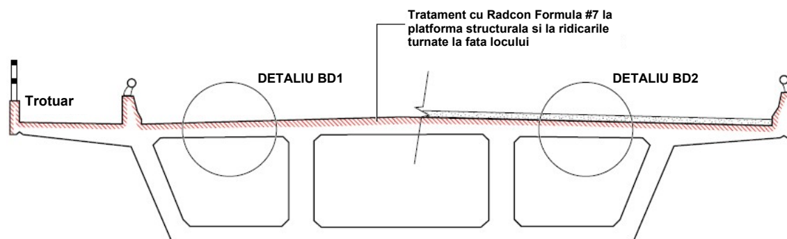
SECTIUNE TIPICA PRINTR-UN POD RUTIER
