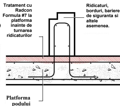
DETALIU BM1 Ridicatura turnata ulterior
