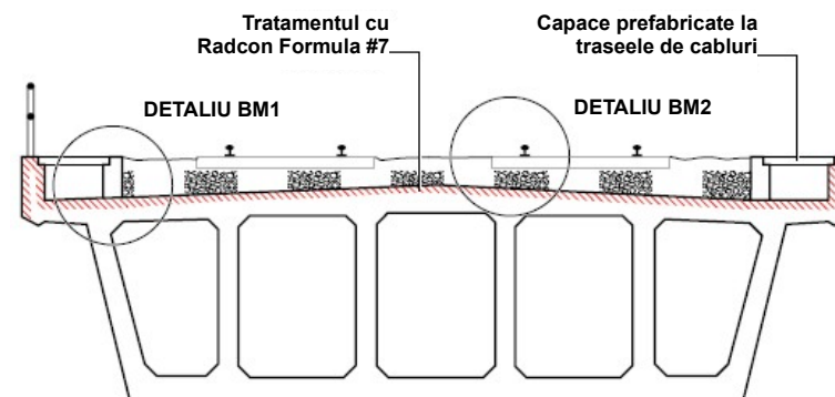
SECTIUNE TIPICA PRINTR-UN POD FERUVIAR
