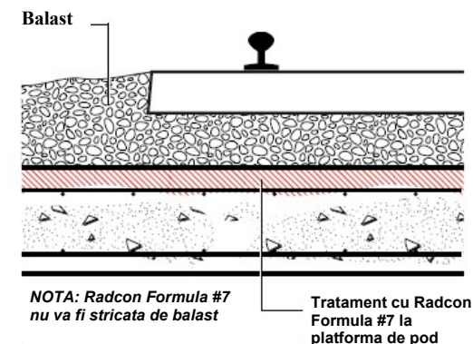
DETALIU BM2 Strat de balast
